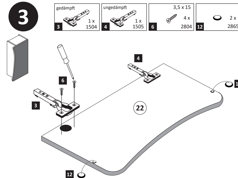
Scharnieransichten von unten
